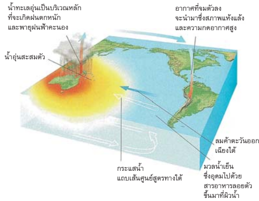
ภาพที่ 1 แผนภาพแสดงปีปกติ (และปีที่เกิดลานีญา)
