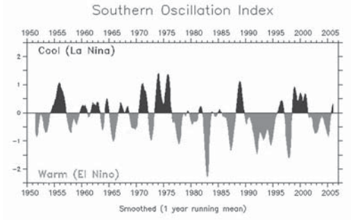
ดัชนี SOI ในช่วงปี ค.ศ. 1950-2005
