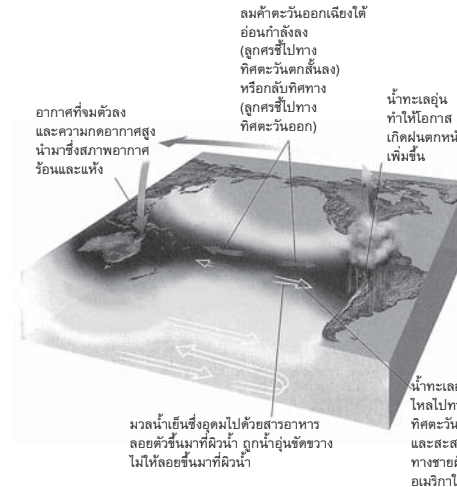
ภาพที่ 2 แผนภาพแสดงปีที่เกิดเอลนีโญ
